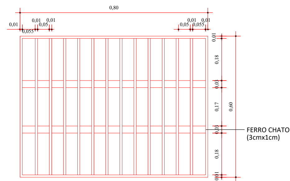
PLANTA - GRELHA
