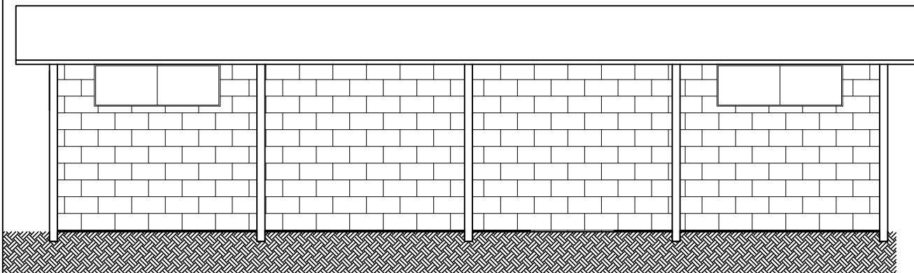
FACHADA LATERAL
